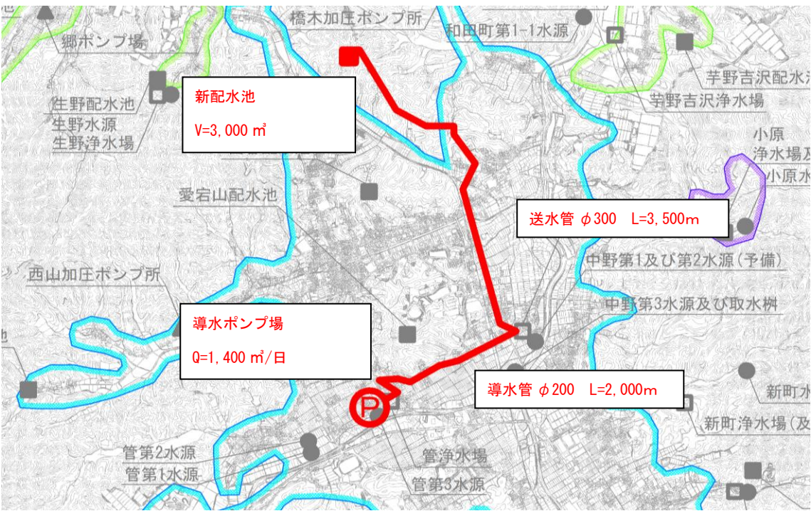
図 2-7 整備計画図 (中野浄水場系)
