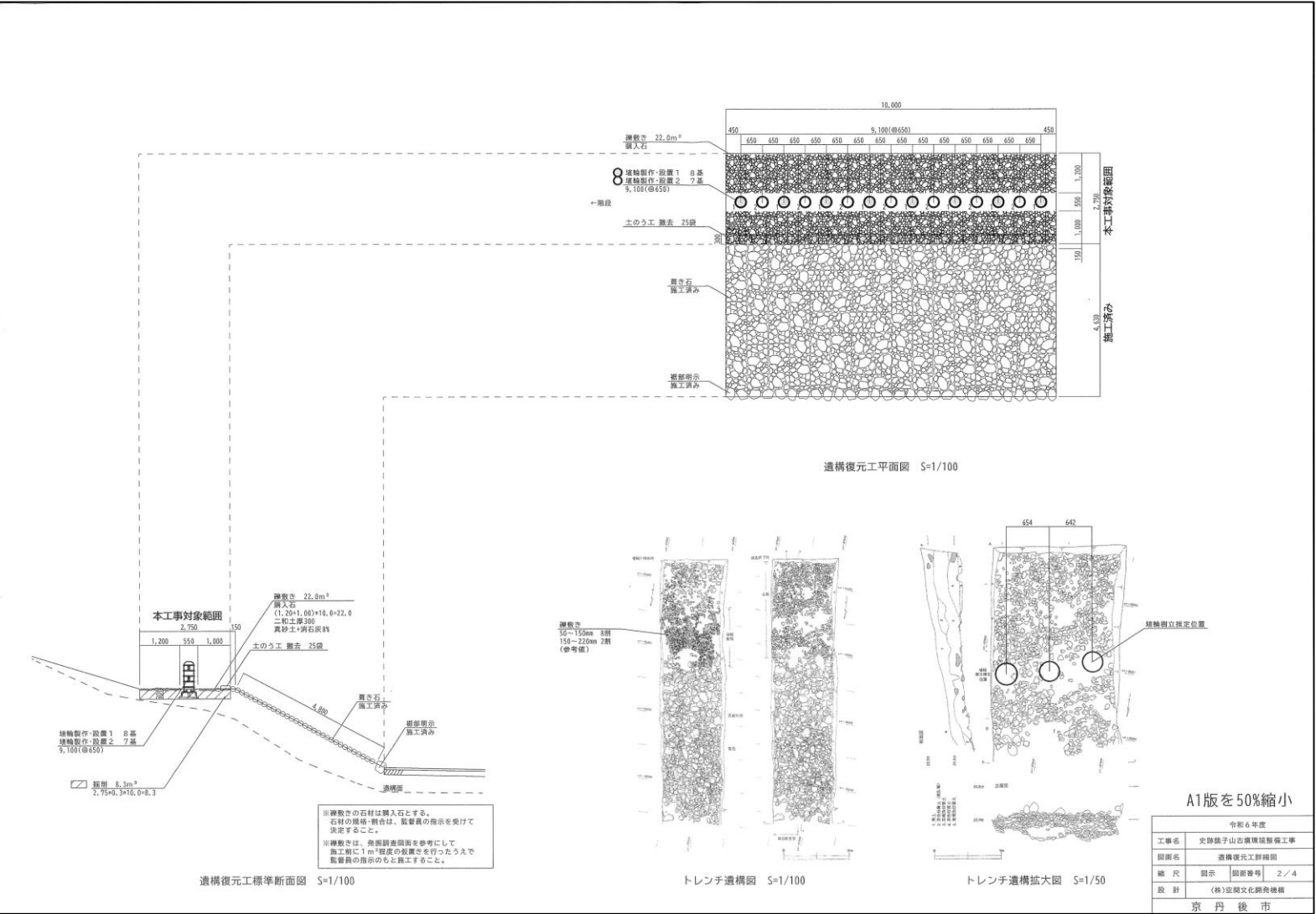
埴輪設置位置・礫敷詳細図
