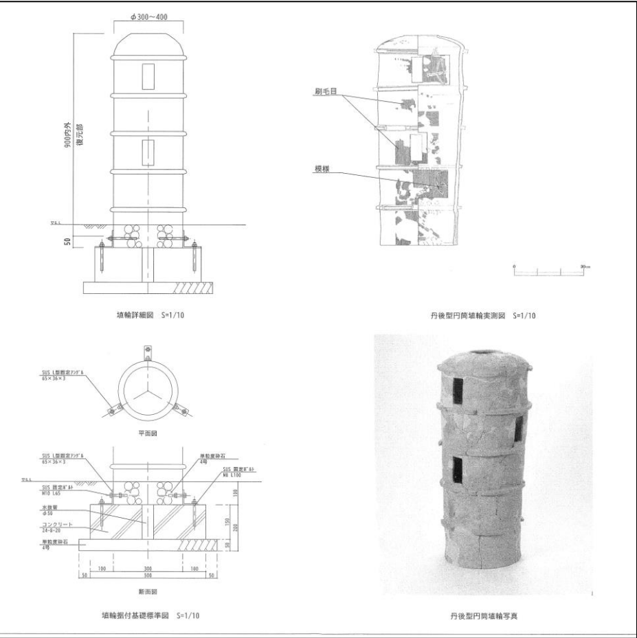
復元埴輪工詳細図
