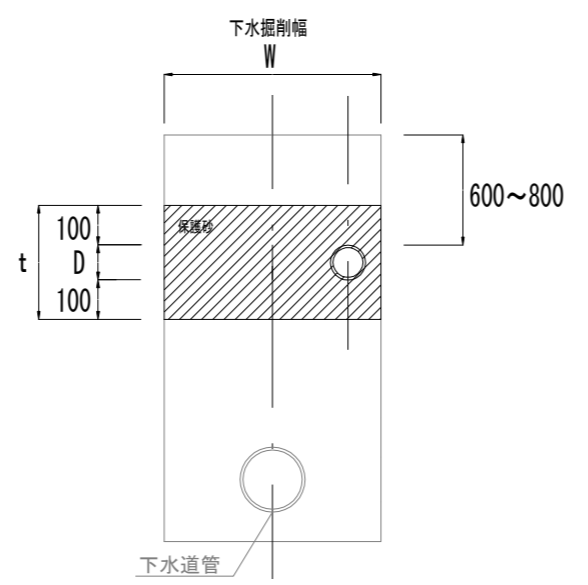
同時埋設工
