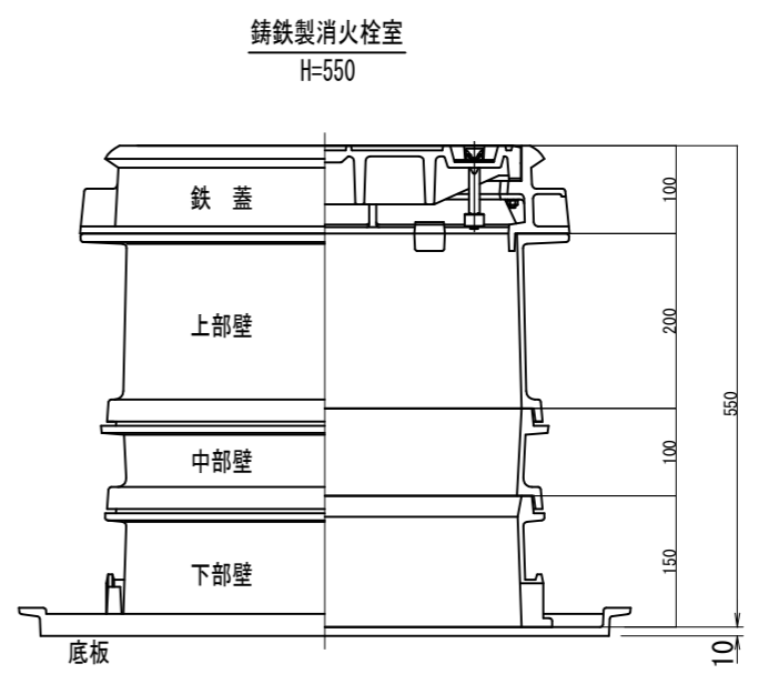
各種標準図 1:5
