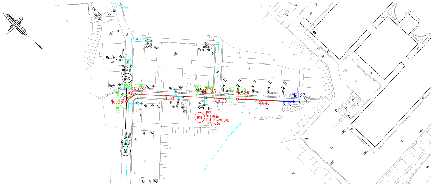
平面図 1:500
