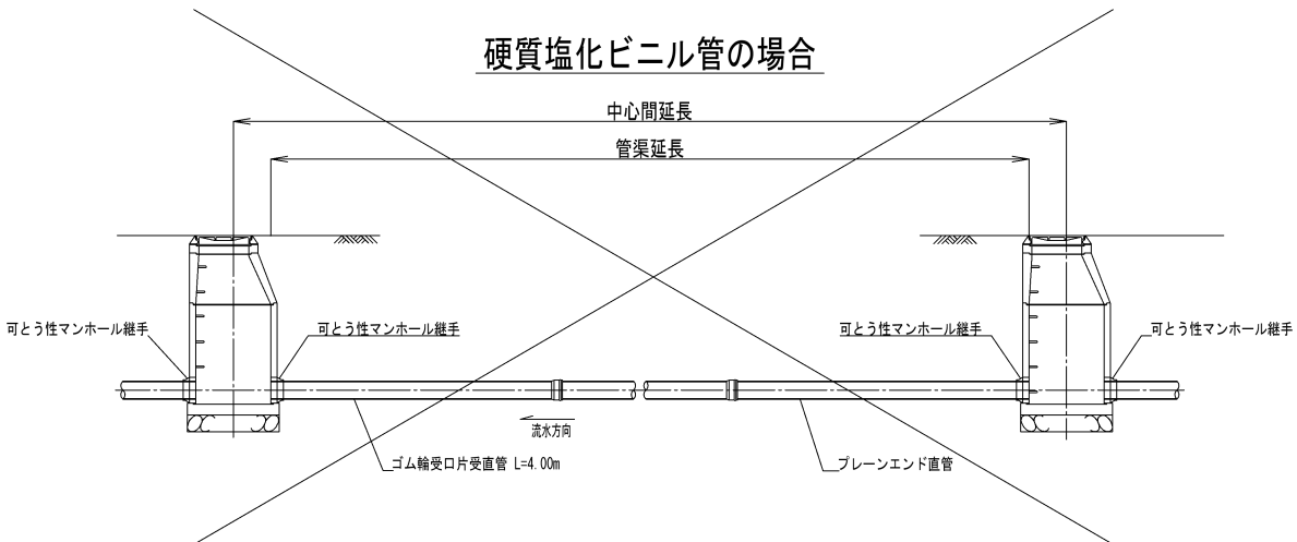
本管布設標準図 S=1:100
