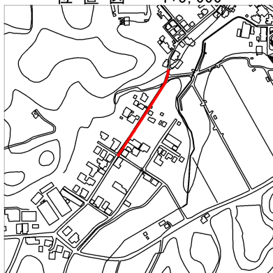
位置図 1:5,000
