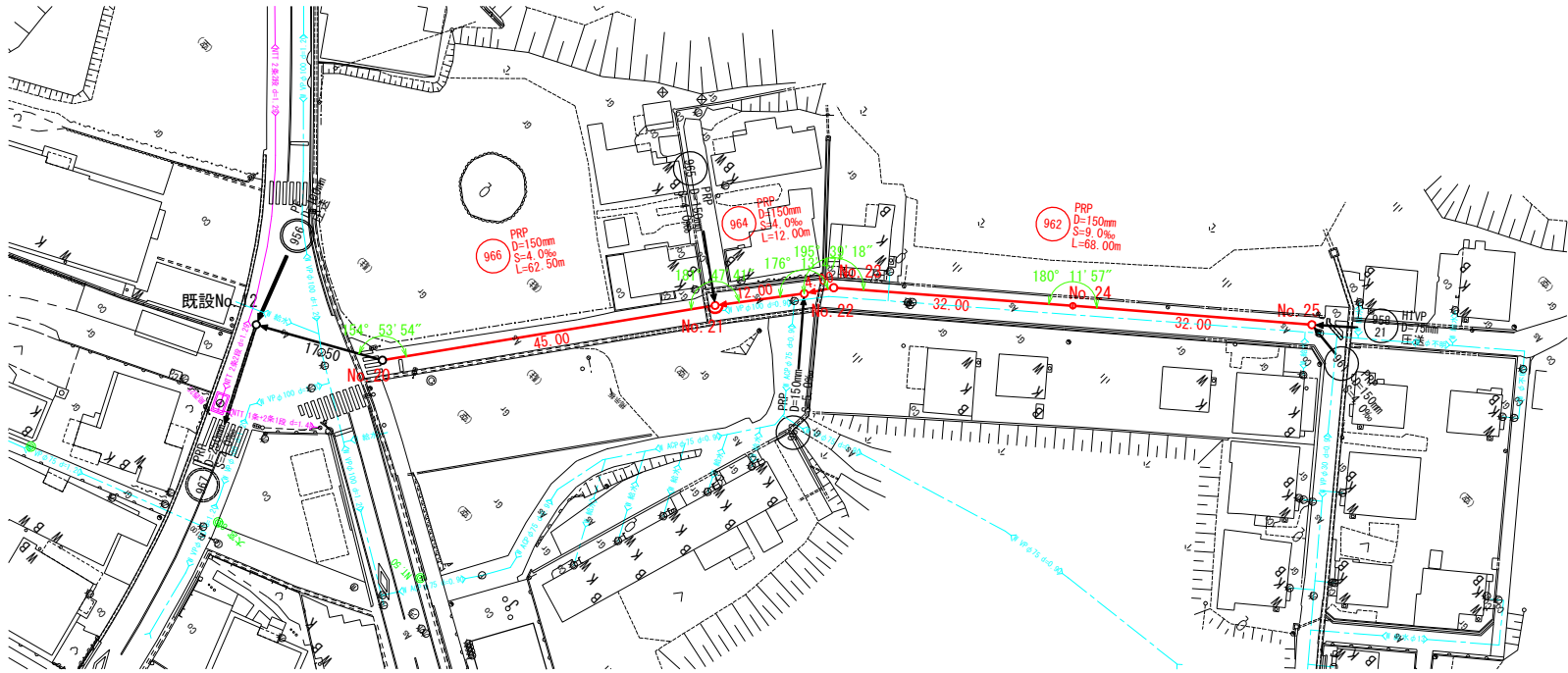
平面図 1:500
