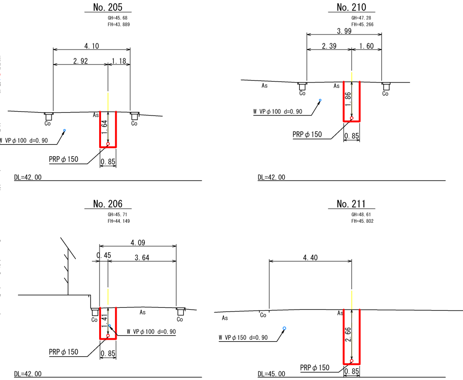
断面図 1:100
