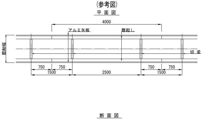
アルミ矢板土留工標準図 S=1:80
