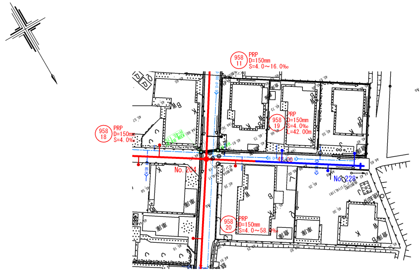
平面図 1:500
