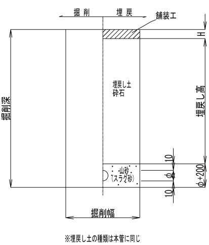
取付管土工定規図 S=1:60
