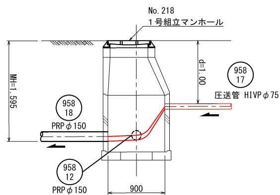
吐出部 詳細図 S=1:30
