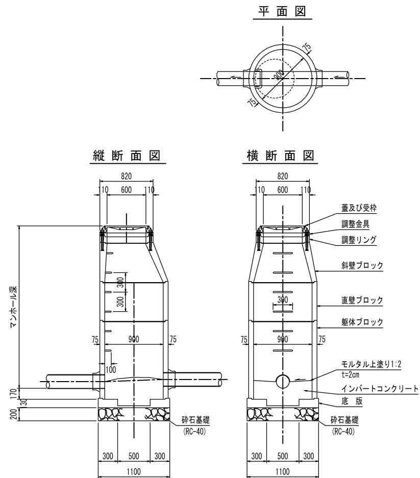
1号組立マンホール S=1:30
