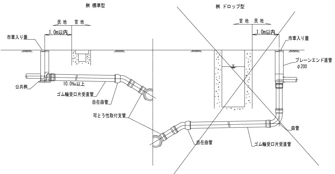
取付管布設標準図 S=1:60
