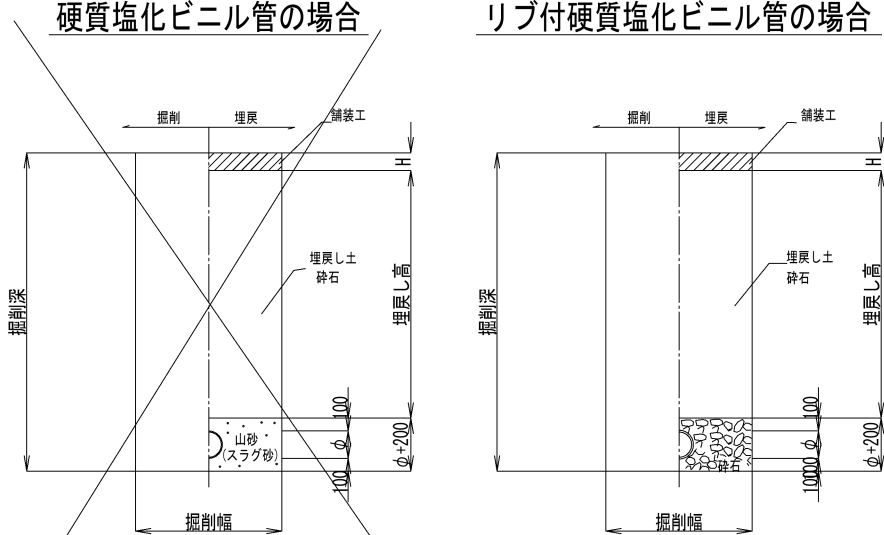
建込み簡易土留 使用区分
