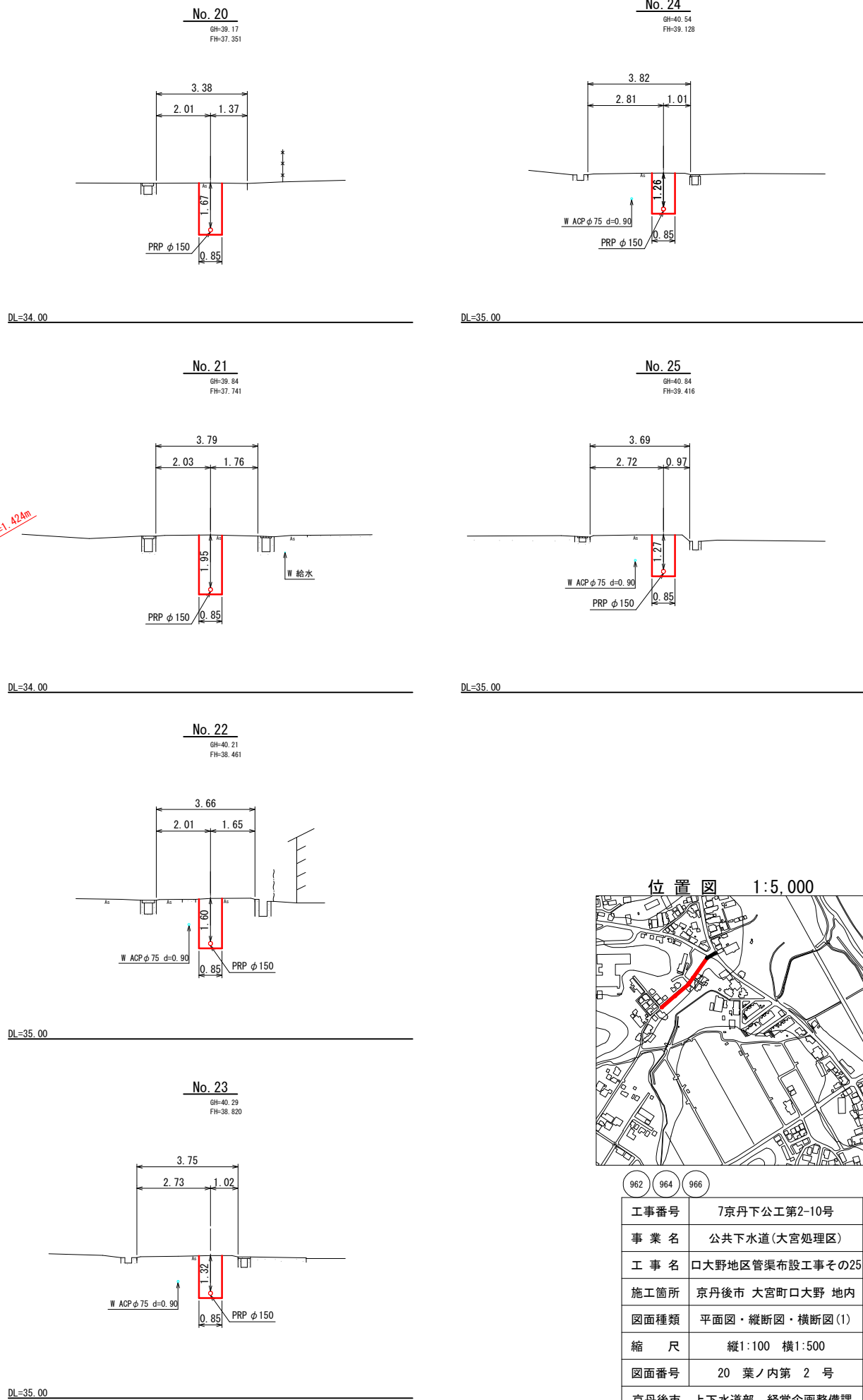
断面図 1:100
