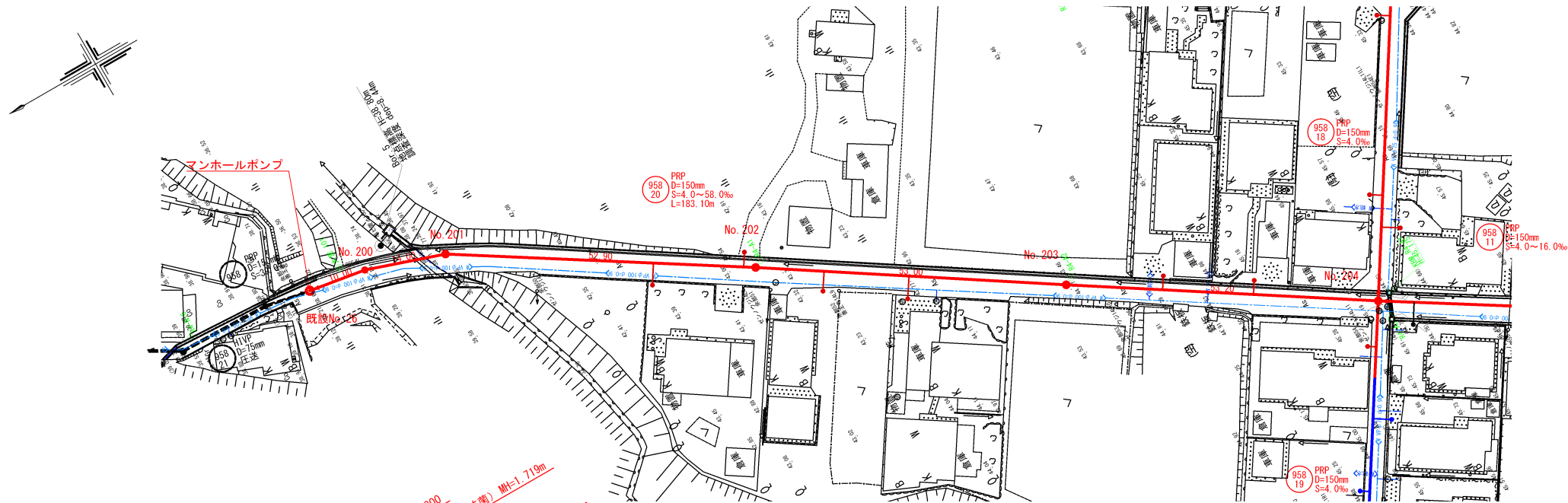
平面図 1:500
