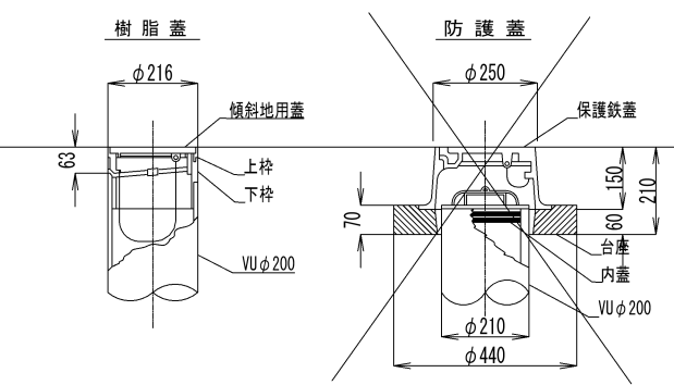
蓋取付詳細図 S=1:20
