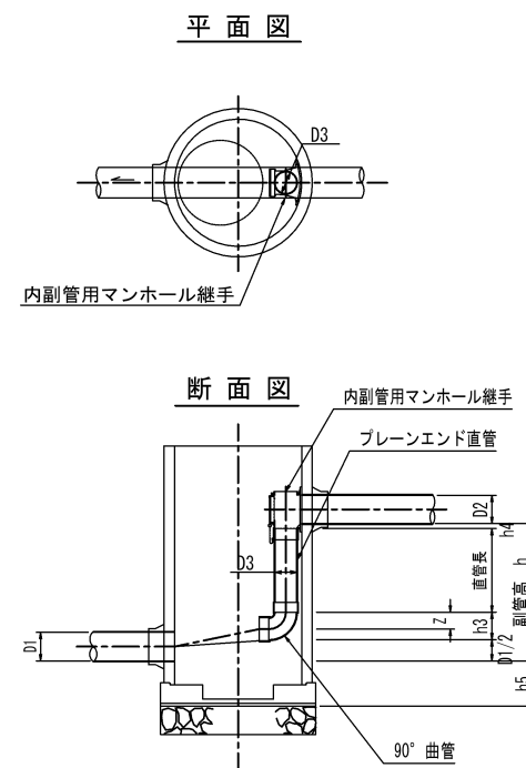
副管標準図 S=1:30
