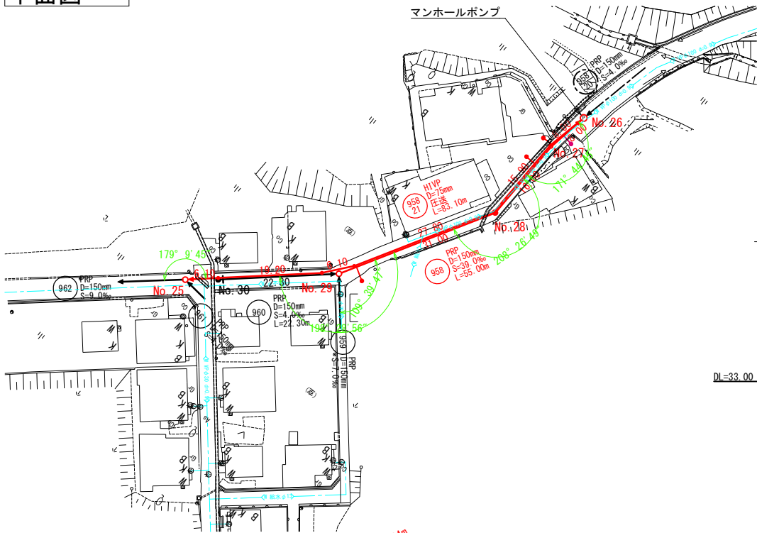
平面図 1:500
