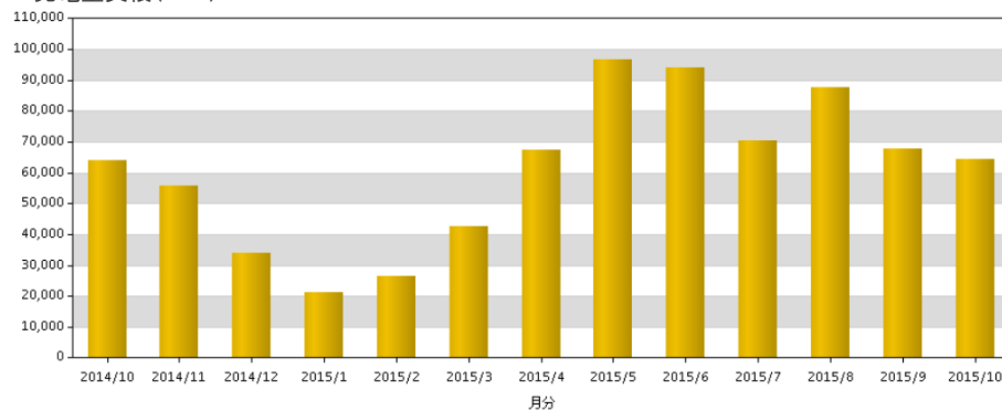
発電量実績(kWh)
