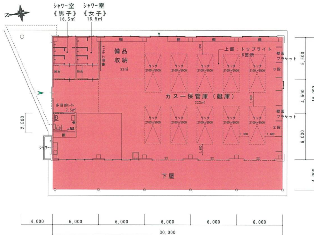
1 階平面図 1:200
