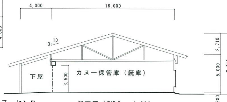
カヌーセンター 断面図《W造》 1:200
