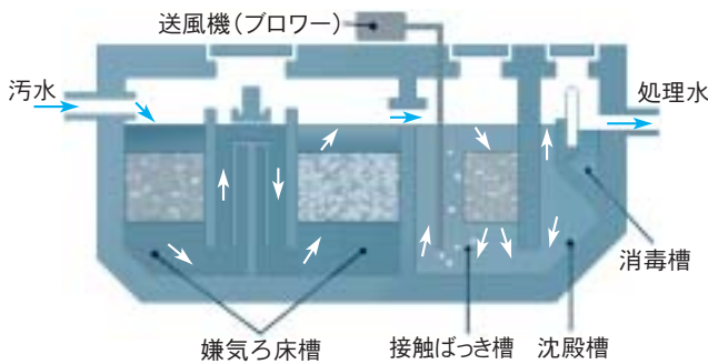
◎合併浄化槽の仕組み
