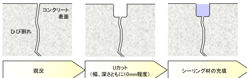
コーキングガンを使用した シーリング材充填
