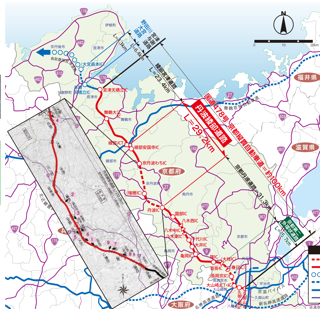
1 改良工事(京丹波町中台地内、平成23年7月撮影) 2 改良工事(京丹波町栗野地内、平成23年4月撮影) 3 改良工事(京丹波町井脇地内、平成23年4月撮影) 4 才原高架橋橋梁工事(京丹波町才原地内、平成23年4月撮影) 5 大朴川橋橋梁工事(京丹波町大朴(おぼそ)地内、平成23年3月撮影) 6 松山高架橋橋梁工事(京丹波町大朴地内、平成23年7月撮影) 7 丹波第一トンネル工事(京丹波町森地内、平成23年4月撮影) 8 曾根川橋橋梁工事(京丹波町森地内、平成23年7月撮影) 9 丹波第一トンネル坑口から丹波第二トンネル坑口を望む、平成23年7月撮影
