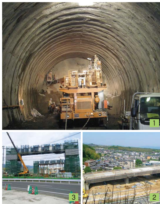
1 西山トンネル(仮称)奥海印寺工区・トンネル掘削工事(長岡京市奥海印寺地内、平成23年4月撮影) 2 沓掛高架橋(仮称)橋梁工事(京都市西京区大枝沓掛町地内、平成23年6月撮影) 3 長岡京第3高架橋(仮称)橋梁工事(長岡京市下海印寺地内、平成23年6月撮影)
