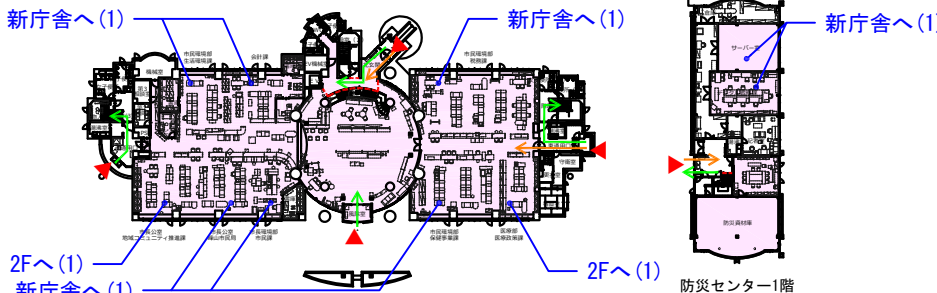
1階平面図
