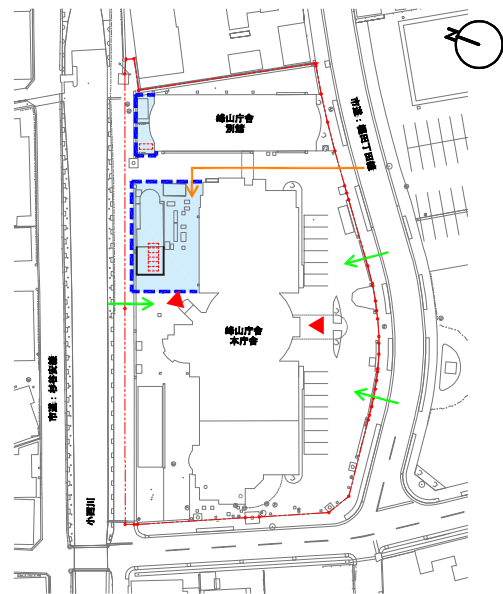
配置図
