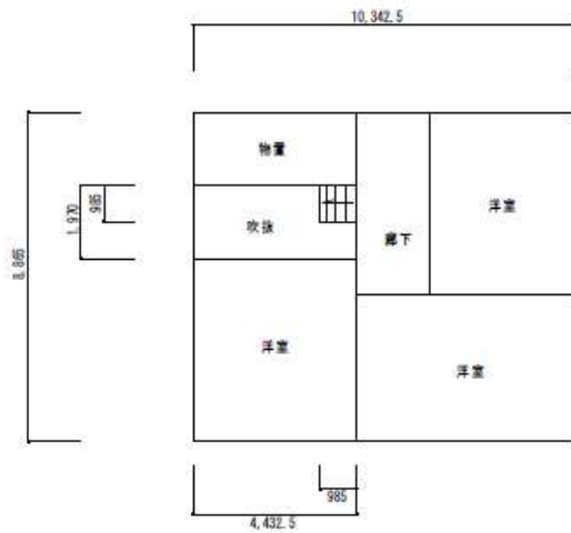
2階 平面図
