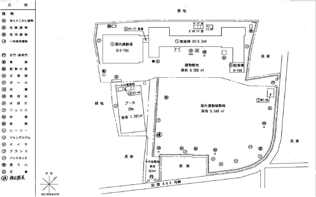
配置図
