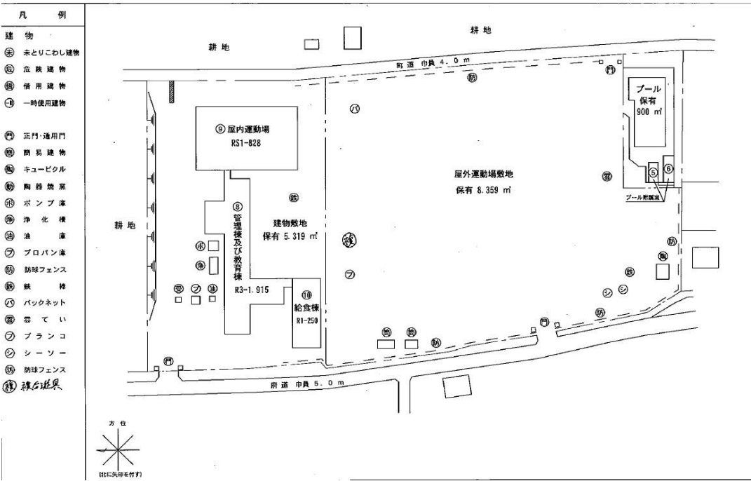
配置図
