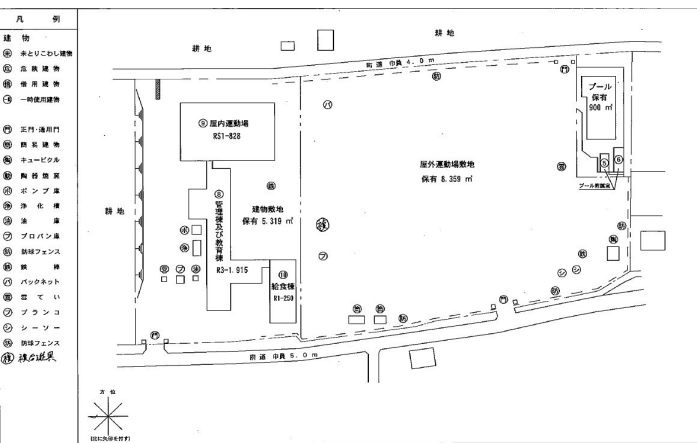
配置図
