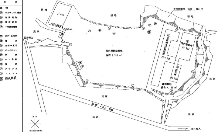
配置図
