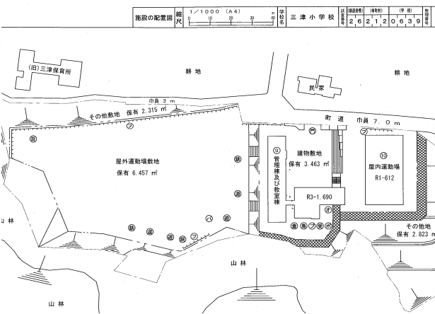
配置図
